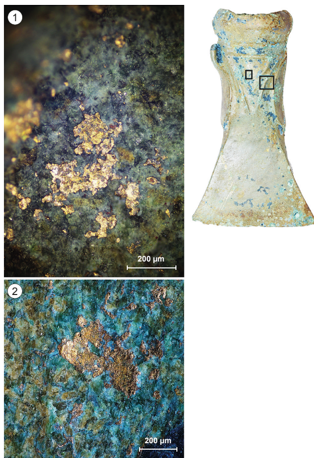
Obr. 16. Vrstvičky kovového lesku na povrchu sekerky inv. č. A 31662/2 (obr. 5: A). 1 – Optický mikroskop pro odražené světlo, zvětšeno 100x; 2 – optodigitální mikroskop, zvětšeno 320x. Foto M. Havlíková.
